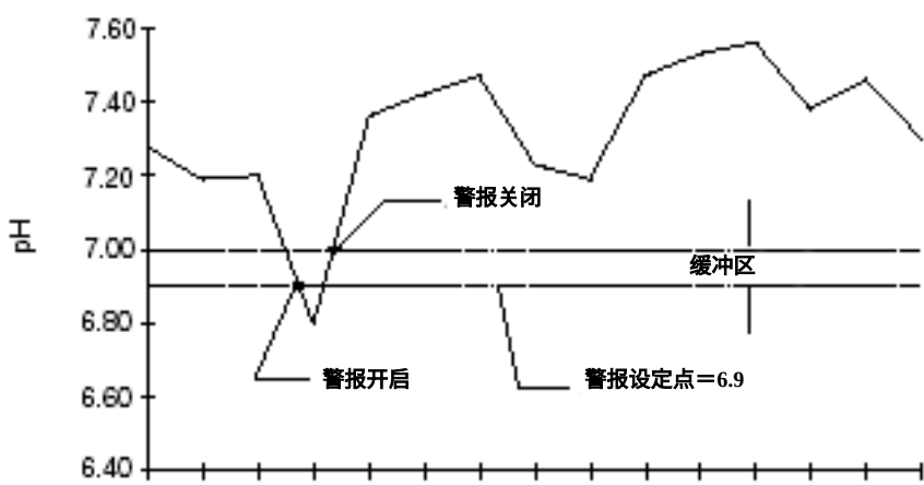
图 56 缓冲区定义
