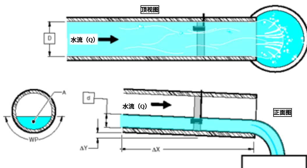
图 55 圆形管道
